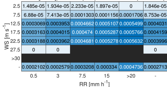
F/R [1/mm], ASPIRE (LES) GEHALX 2022 (n = 77626)
