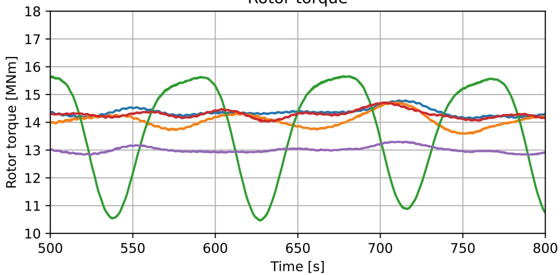
Rotor torque
