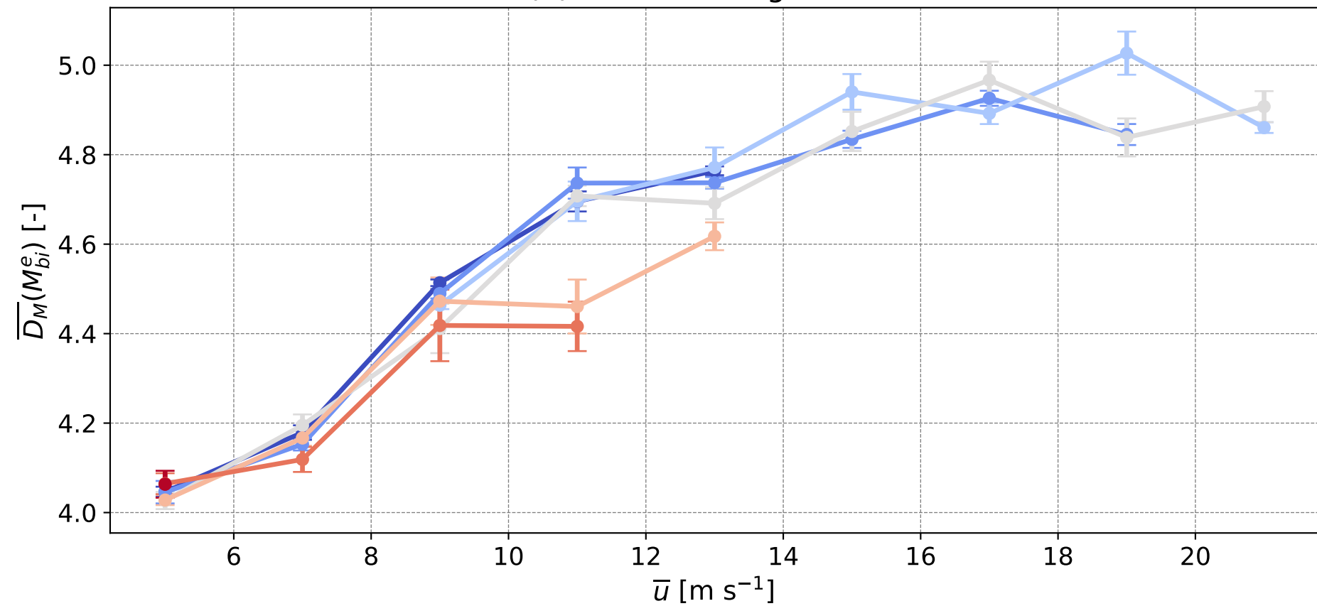
(b) Blade-root Egdewise
