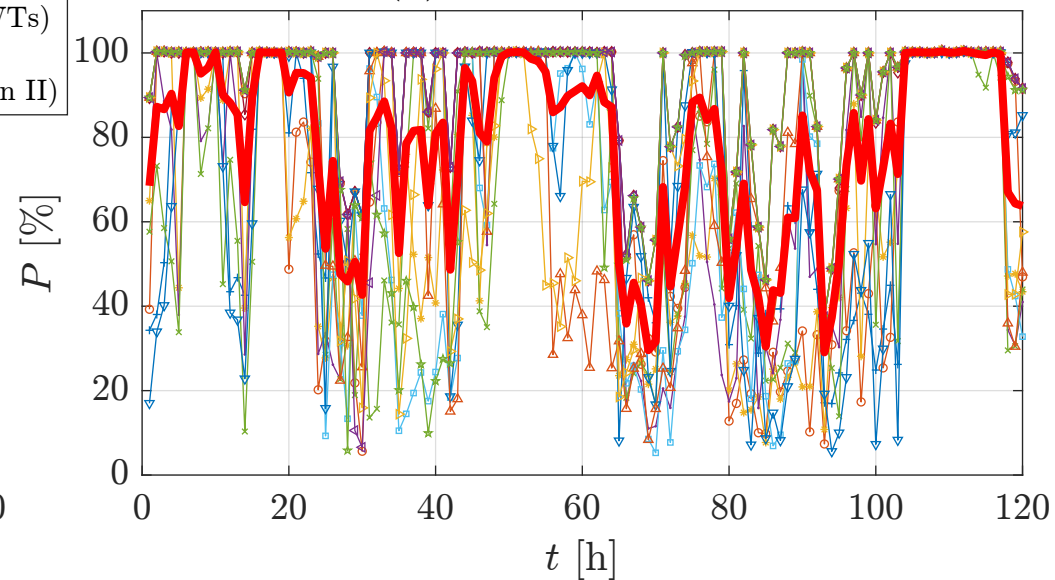
(d) Max. Virtual Inertia for P_{\text{set}} = 1
