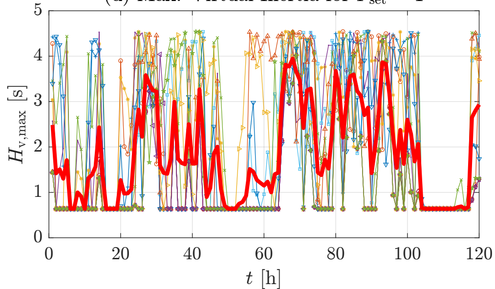
(d) Max. Virtual Inertia for P_{\text{set}} = 1
