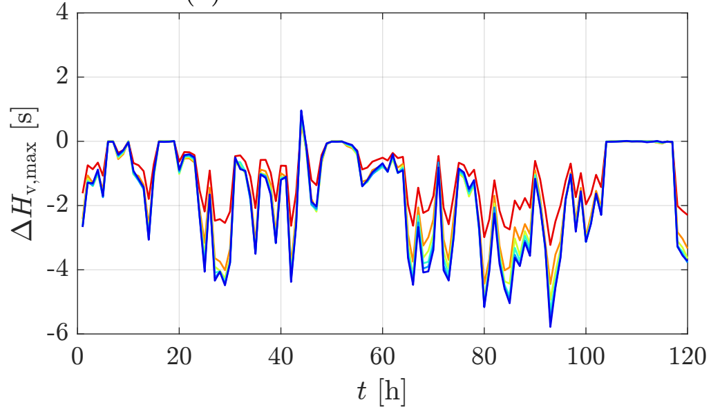
(d) “Comb Min”-Forecast Error
