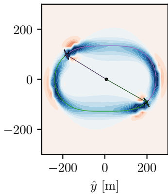
Vortex-loop model
