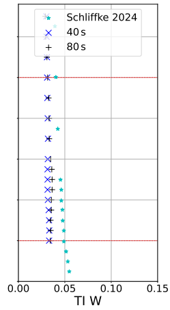
(d) Inlet I_W
