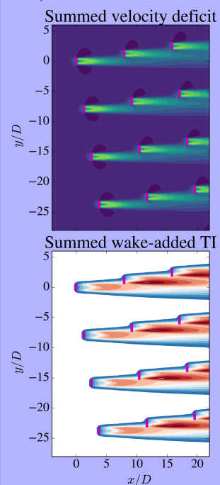
m) All2AllIterative
