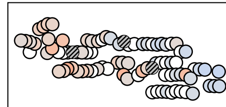
ID 15: LLNL WRF+LES (mesoscale+LES)
