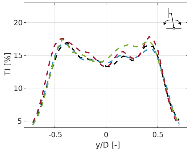
ALM URANS POLIMI
