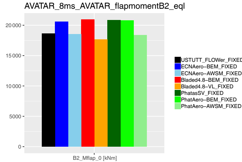
(d) Fatigue equivalent flapwise blade root moment
