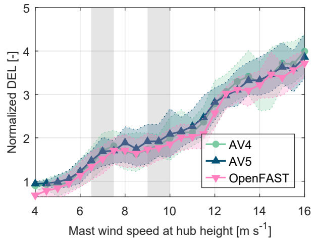
(d) Blade-root flapwise bending moment
