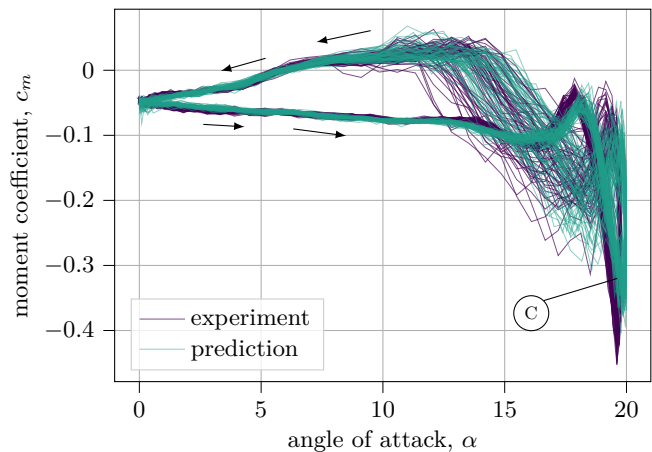
(d) Moment DTW + EMD score = 1.40
