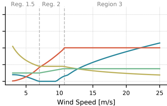
IEA 15-MW
