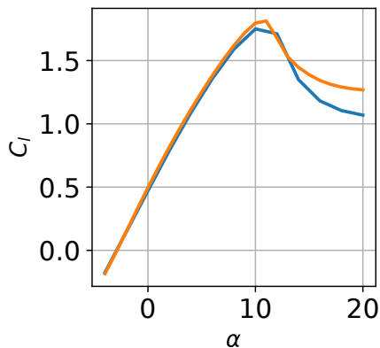
FFA-W3-360GF
