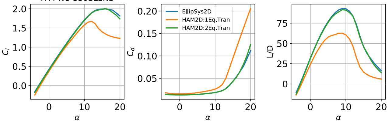
(d) FFA-W3-330BLEND airfoil at Re = 10 \times 10^6
