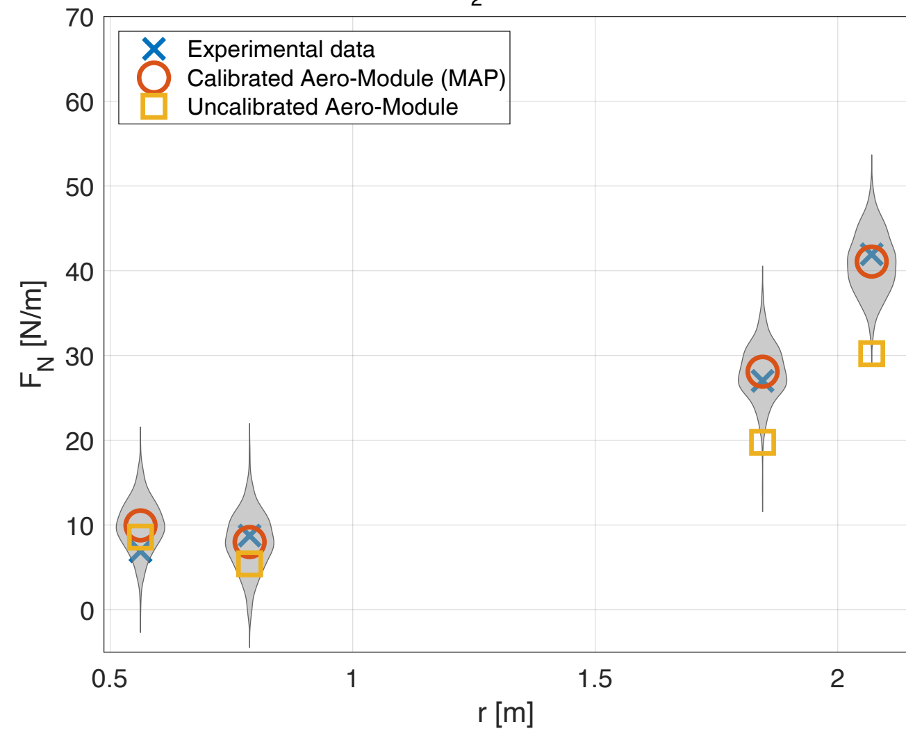
Scenario S_2 (yaw angle 30^\circ )
