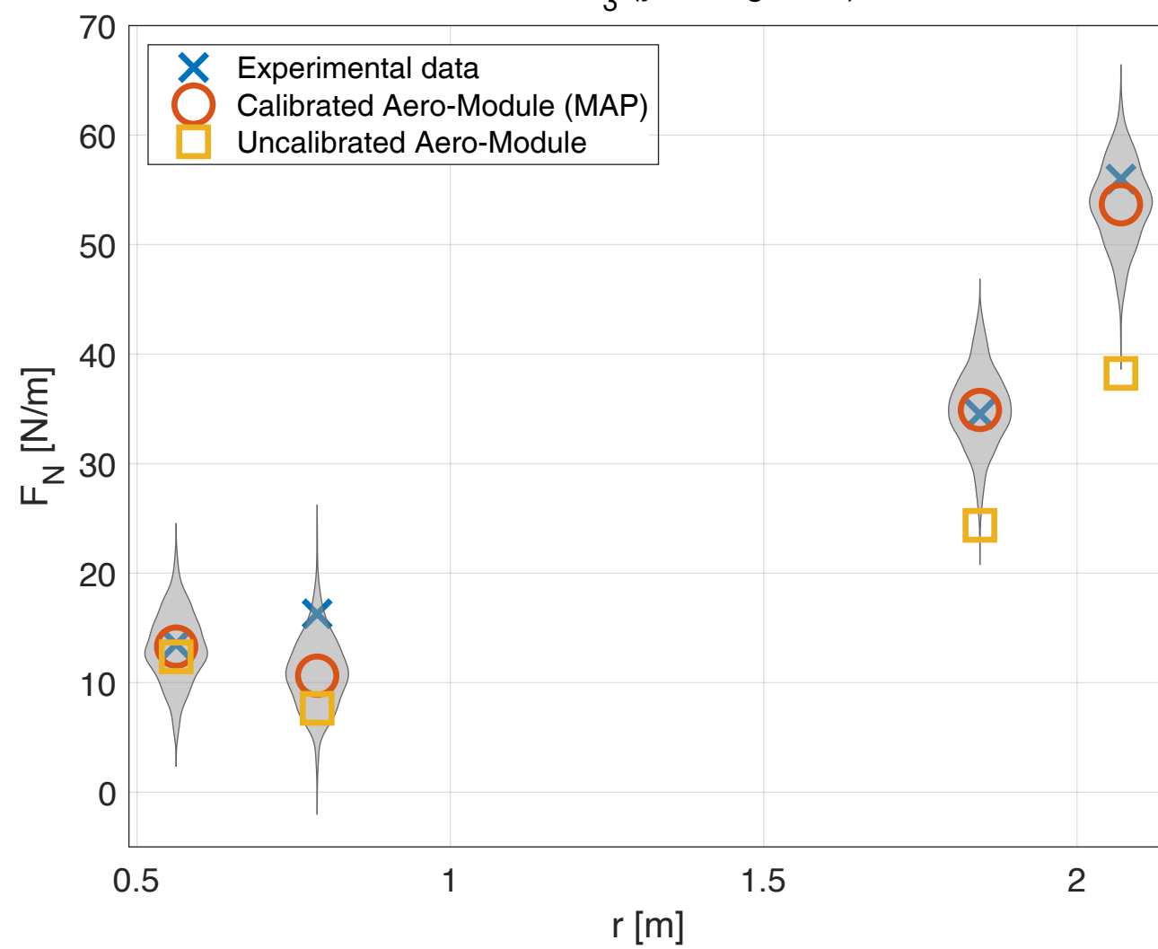
Scenario S_3 (yaw angle 45^\circ )
