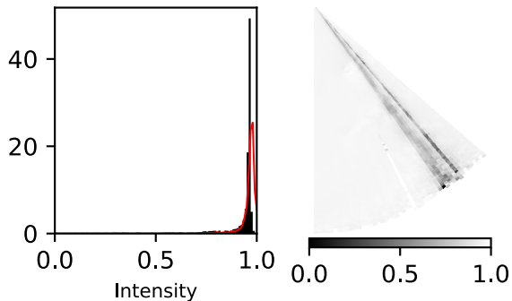
(d) Corrupted
