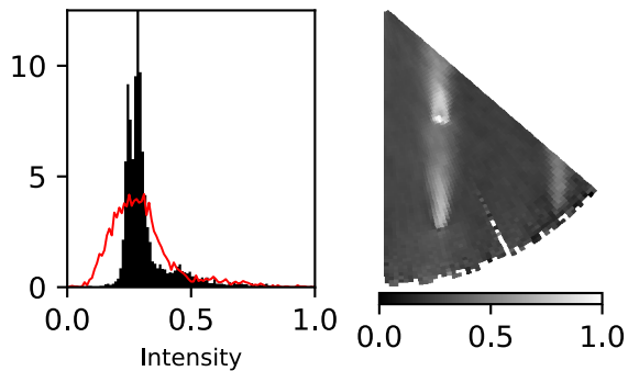
(d) Corrupted
