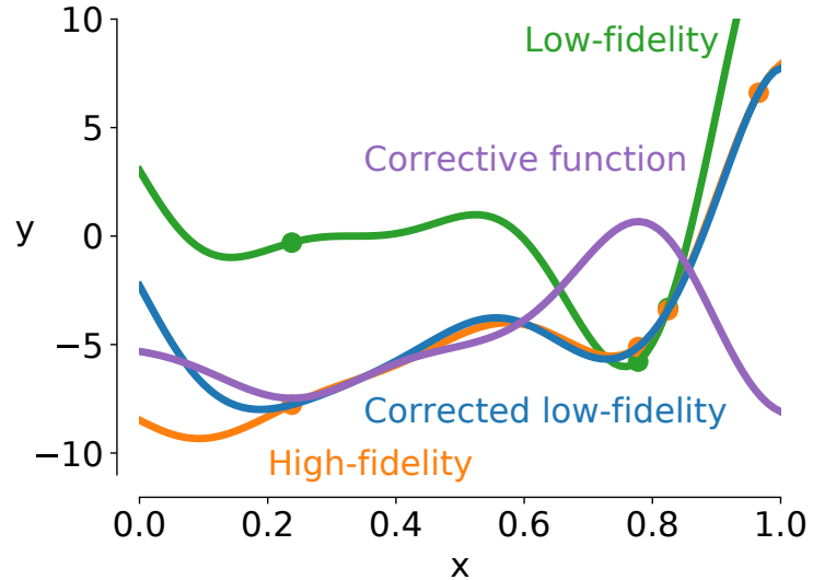
(c) KPLS
