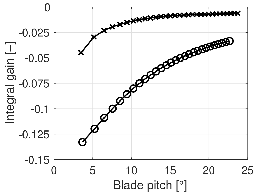
—○— IEA 15 MW (model scale) —×— WTM
