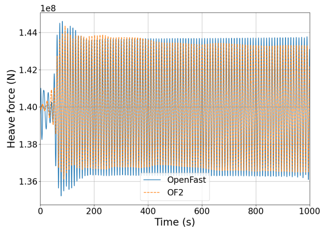
(d) LC 3.1 Heave force
