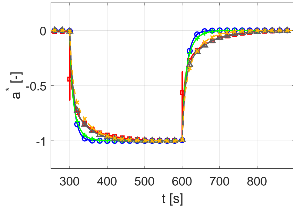
(d) - Normalized Axial induction - r/R = 95\%
