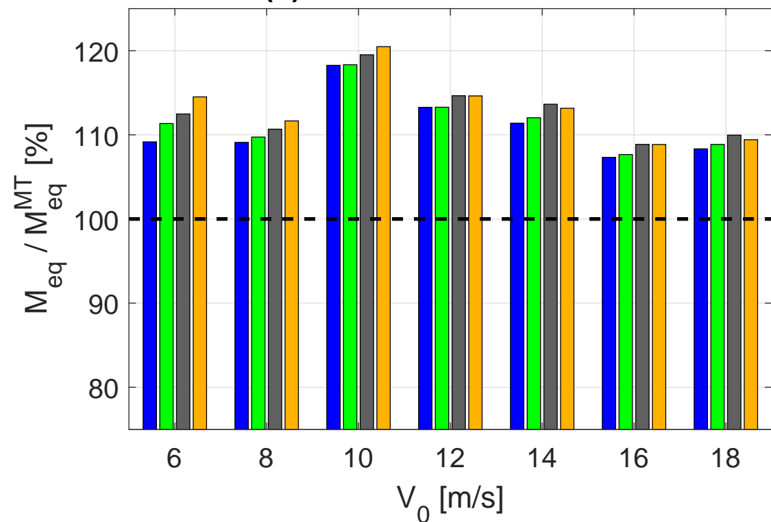
(d) Tower fore-aft moment
