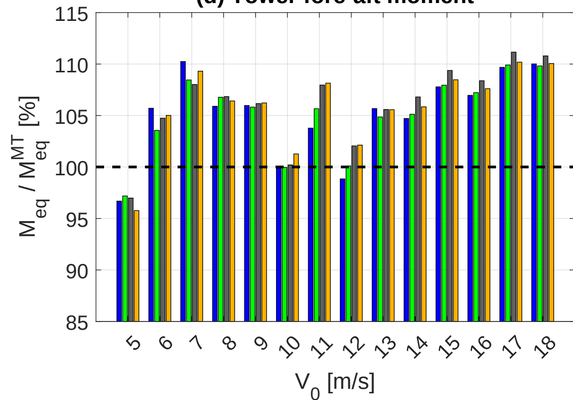
(d) Tower fore-aft moment
