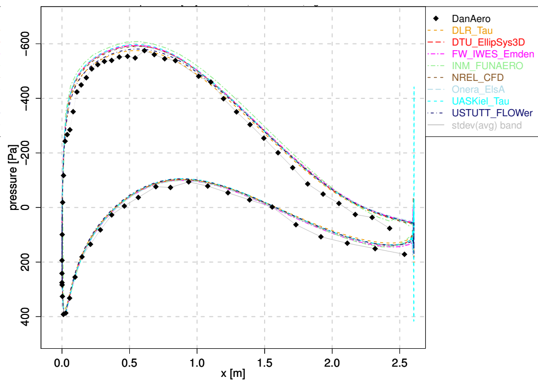
(d) Pressure at r=19.06 m
