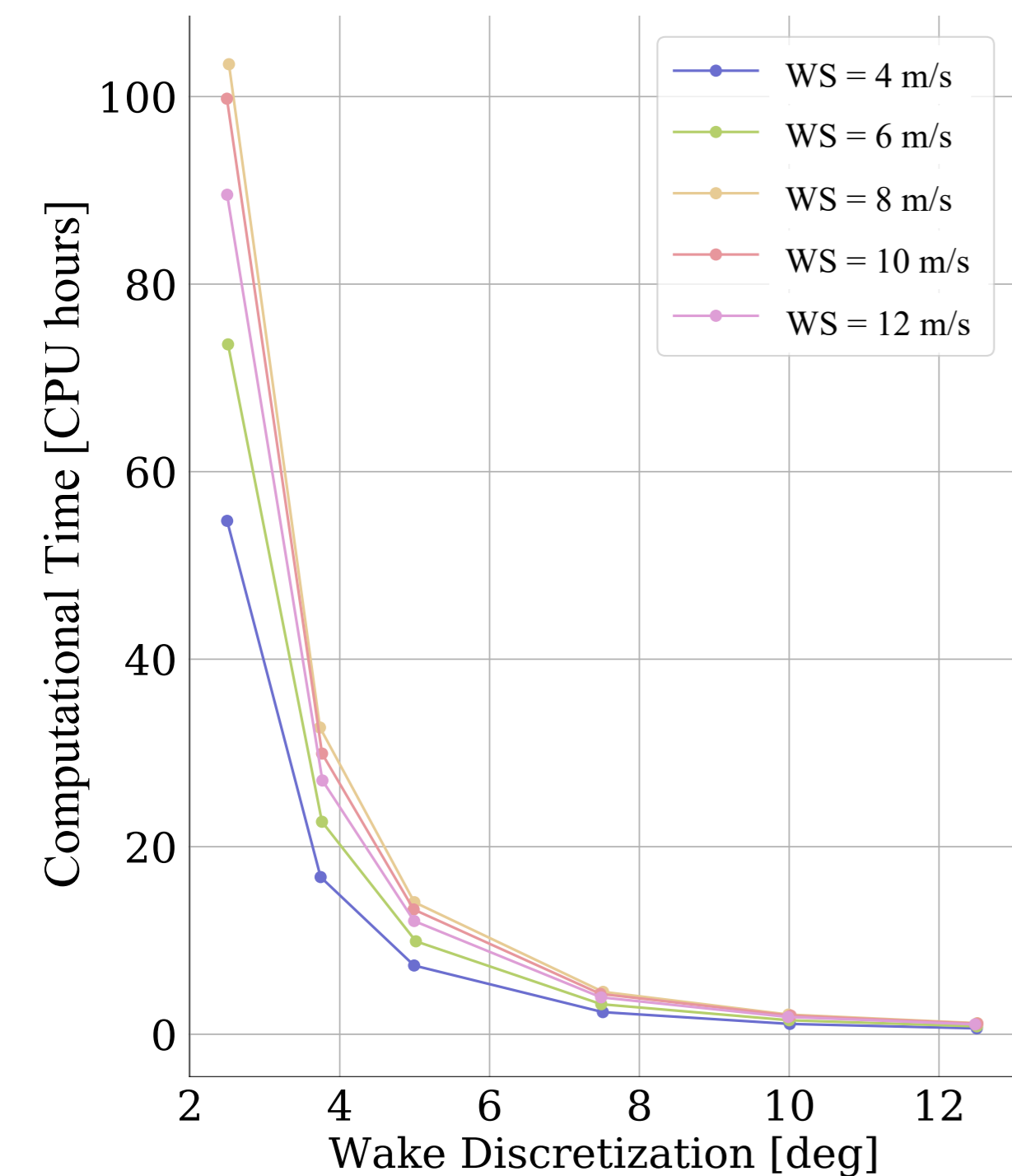
(d) Wake discretization computational time
