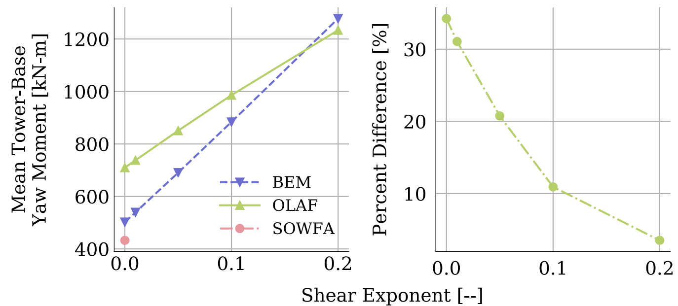
(d) Tower-base yaw moment
