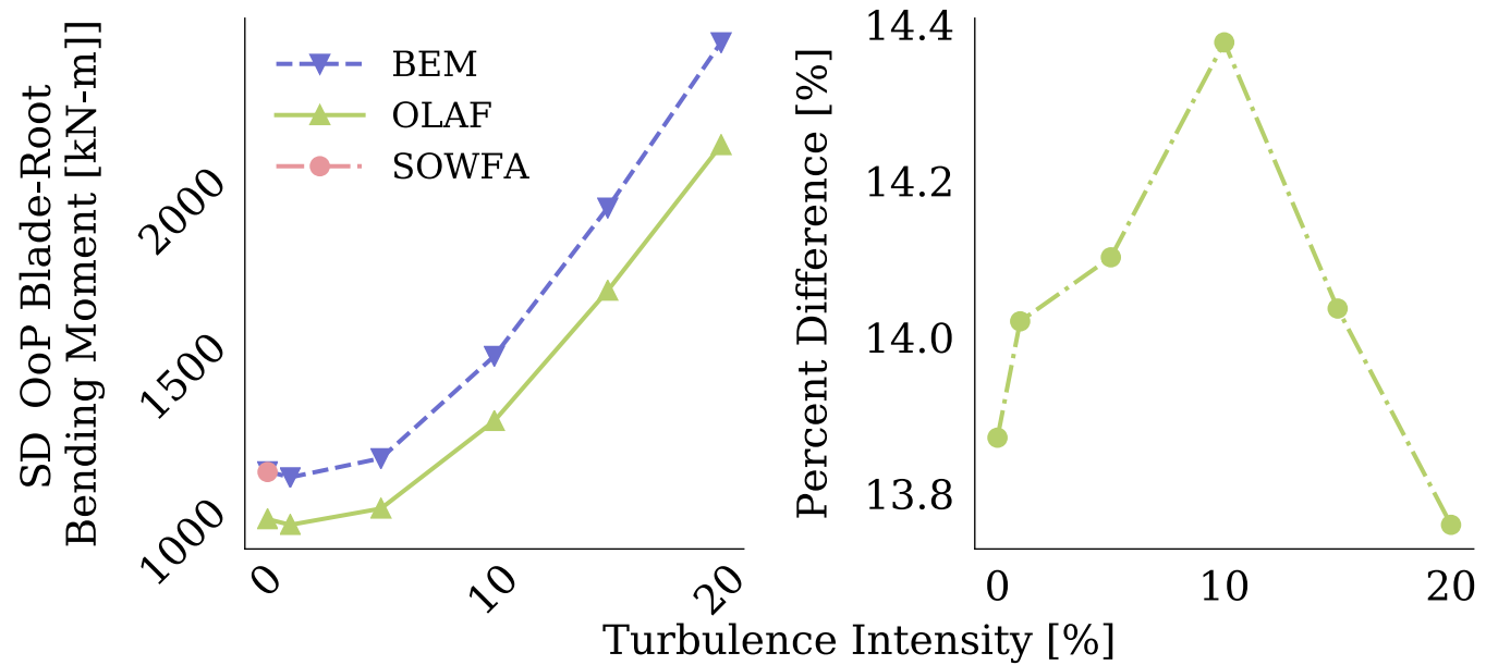
(d) SD out-of-plane blade-root bending moment
