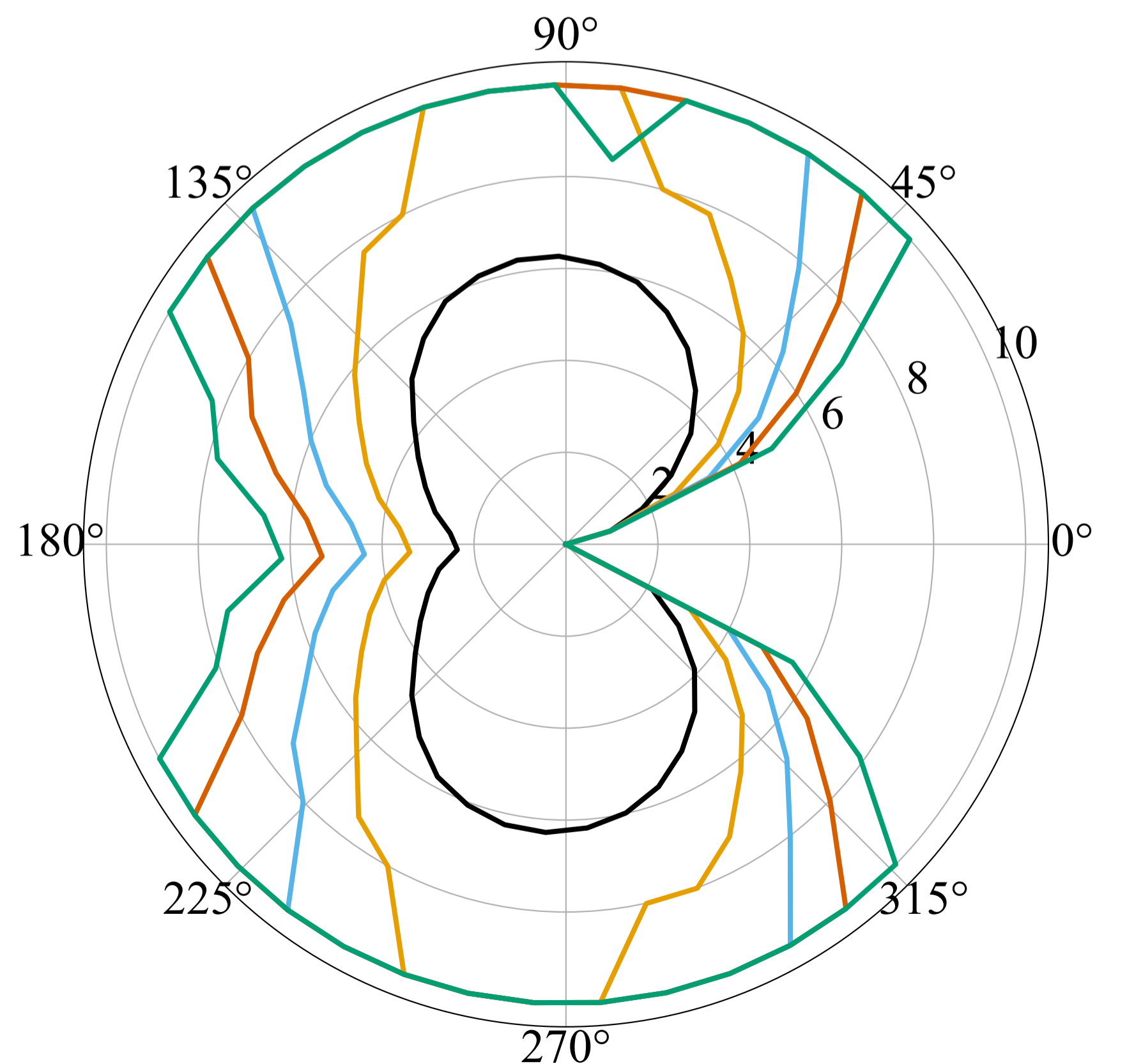
(d) Optimal vessel speed ( V_b , m/s)
