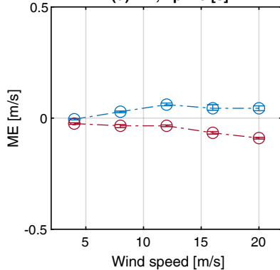
(d) ME, T_p = 6 [s]
