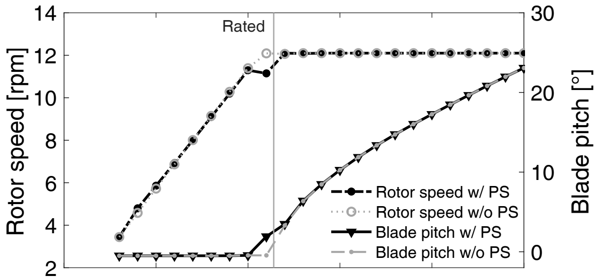
NREL 5 MW
