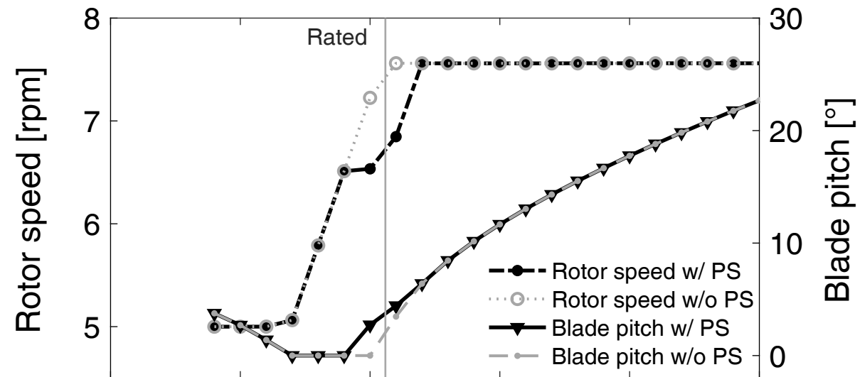
IEA 15 MW
