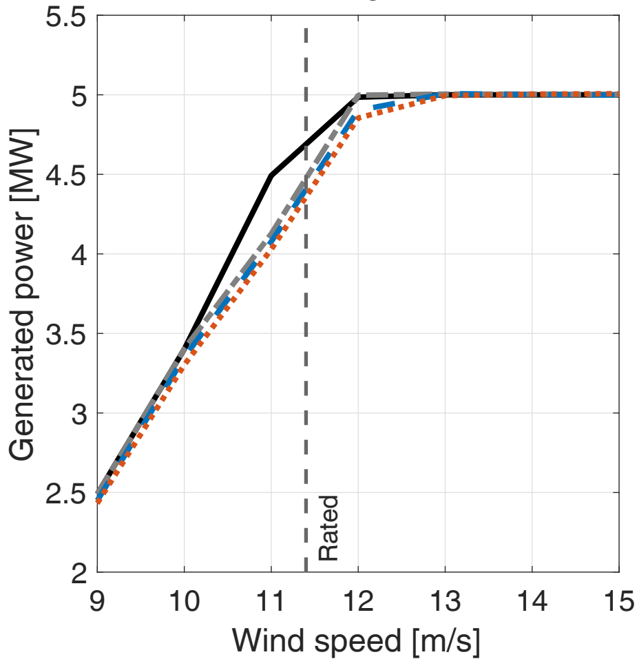
NREL 5 MW
