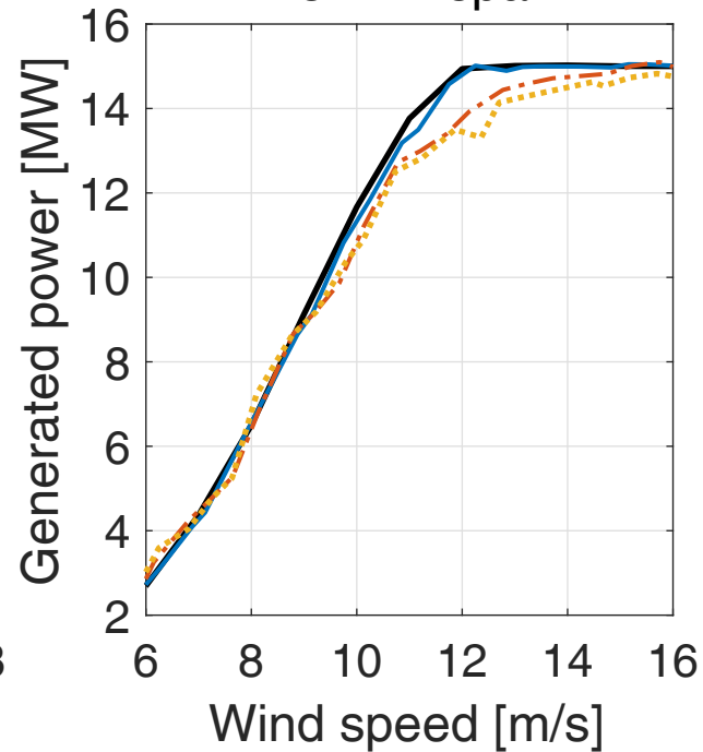
15 MW spar
