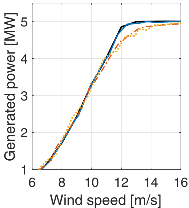
5 MW spar
