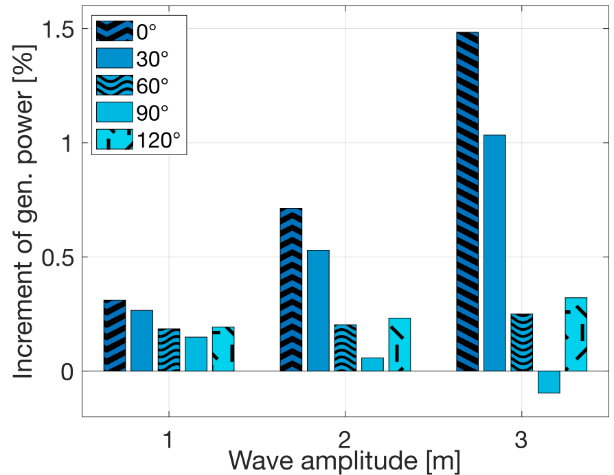
15 MW spar
