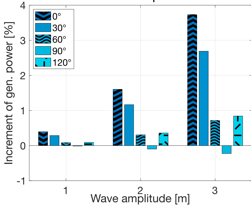
5 MW spar
