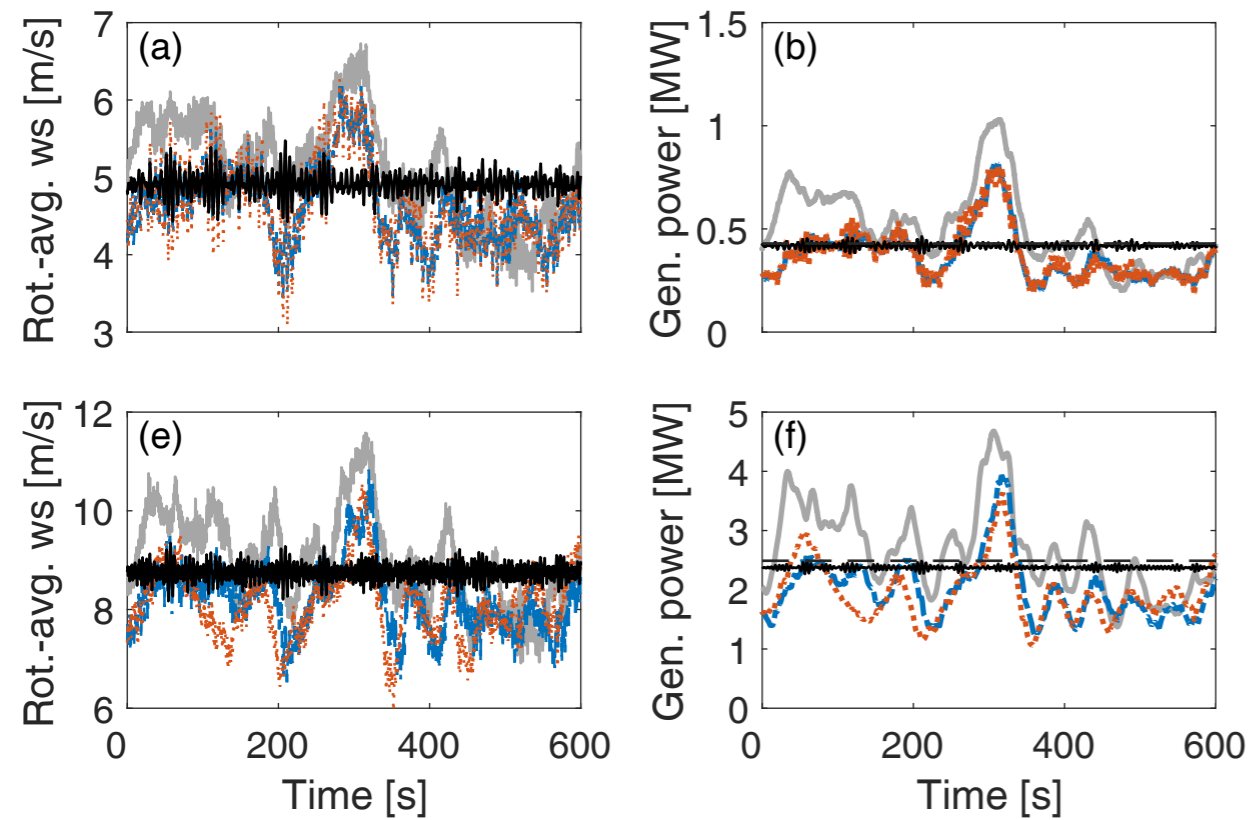
5 MW spar
