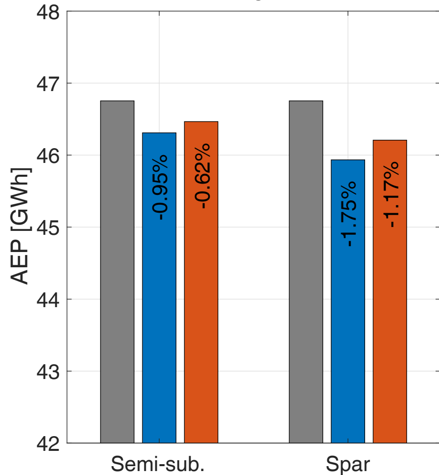
IEA 15 MW
