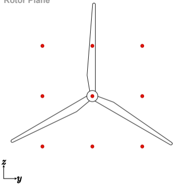
(a) TurbSim output
