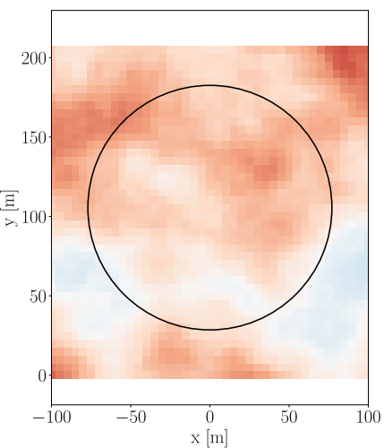
(d) Medium speed - BHawC
