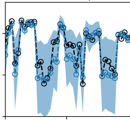
Matérn 3/2
