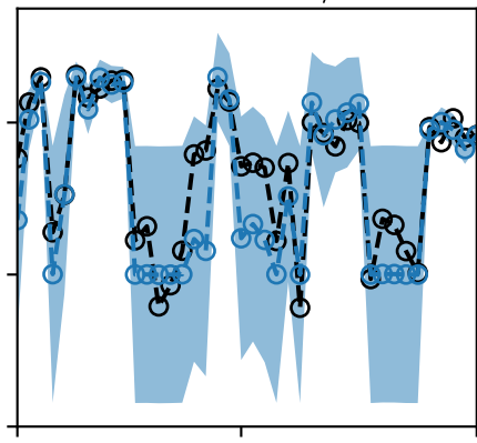
Matérn 5/2
