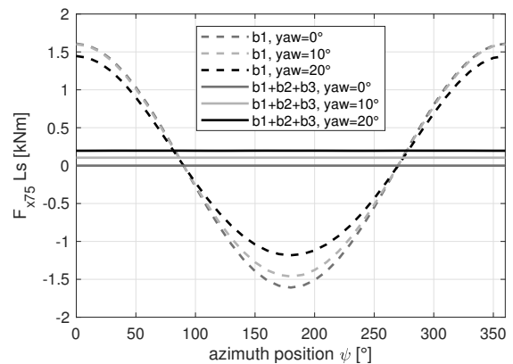
(d) Yaw moment estimate from F_x at R = 75\% .
