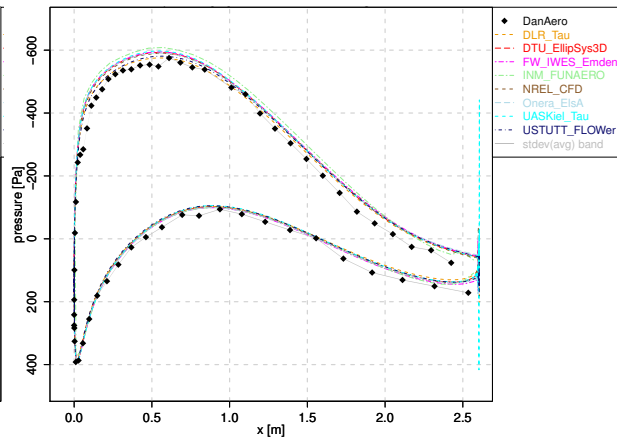
(d) Pressure at r=19.06 m
